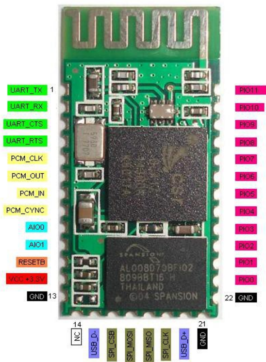
Рис. 3 - Наименование и расположение выводов модуля HC
